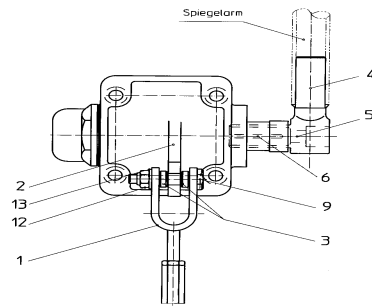
Skizze - Lager
