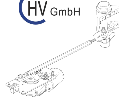
Antrieb – Gestänge - Lager
