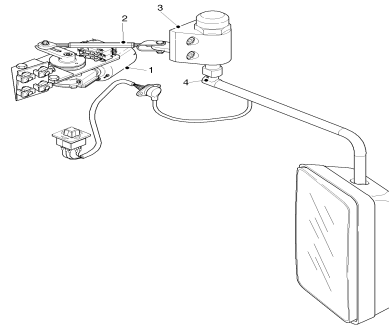
Prinzip – Skizze
